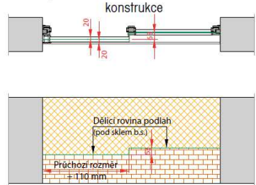
Dveře posuvné s bočním světlíkem – rámová konstrukce
