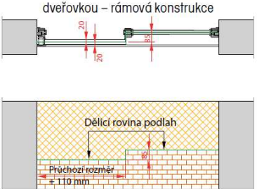
Dveře posuvné s bočním světlíkem a dveřovkou – rámová konstrukce
