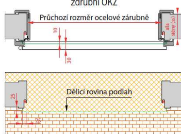
Dveře otočné polodrážkové se zárubní OKZ
