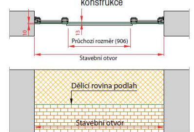
Dveře otočné polodrážkové – rámová konstrukce
