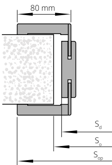
Tunel ZN s obložkami DUO „80“
