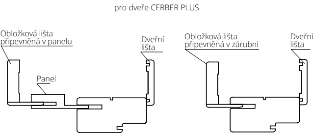
pro dveře CERBER PLUS
