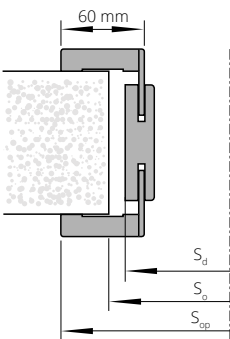
Tunel ZN s obložkami „60“
