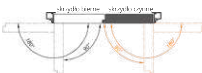
D. Pravé dveře otevírané směrem ven
