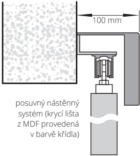
posuvný nástěnný systém s tunelovou zárubní ZN (netýká se systému Premium)
