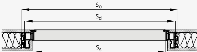
DVEŘE HARMONY INVEST (OTEVÍRÁNÍ DOVNITŘ) ODW
